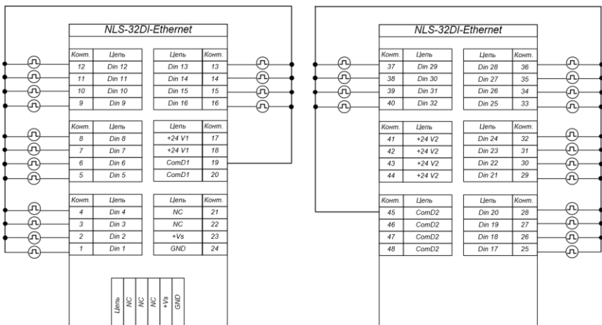
Рис. 4.22. Подсоединение источников сигналов с логическими уровнями
