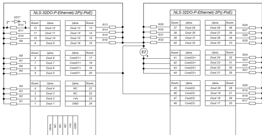
Рис. 4.26. Применение модулей NLS-32DO-P-Ethernet(-PoE), NLS-32DO-P-Ethernet-2P(-PoE) для управления нагрузкой, с питанием от одного внешнего источника
