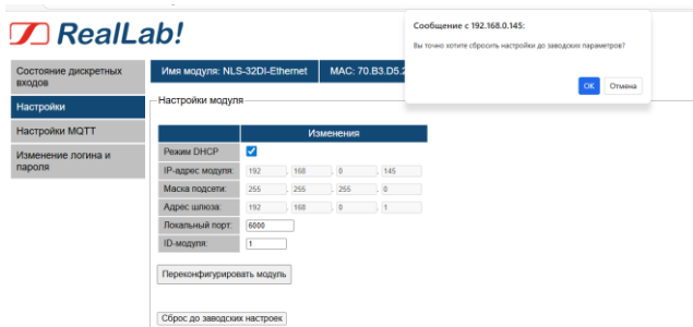
Рис. 4.16. Окно подтверждения сброса настроек
