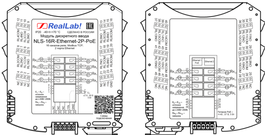
Рис. 1.13. Вид со стороны маркировки на модуль NLS-16R-Ethernet-2P-PoE
