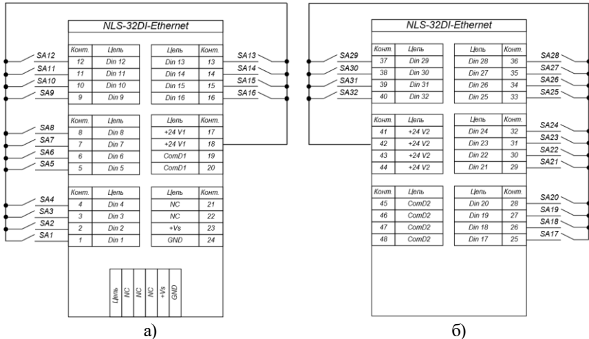
Рис. 4.18. Подсоединение контактов к модулю датчиков типа «Сухой контакт», где:
