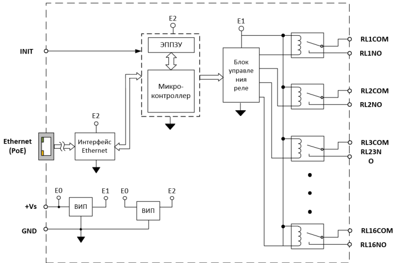
Рис. 3.7. Структурная схема модуля NLS-16R-Ethernet(-PoE) Обозначения: COM - "Common" - "общий", "NO" - "Open" - нормально открытый
