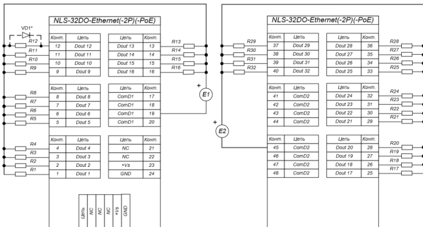
Рис. 4.23. Применение модулей NLS-32DO-Ethernet(-PoE), NLS-32DO-Ethernet-2P(-PoE) для управления нагрузкой, где:
