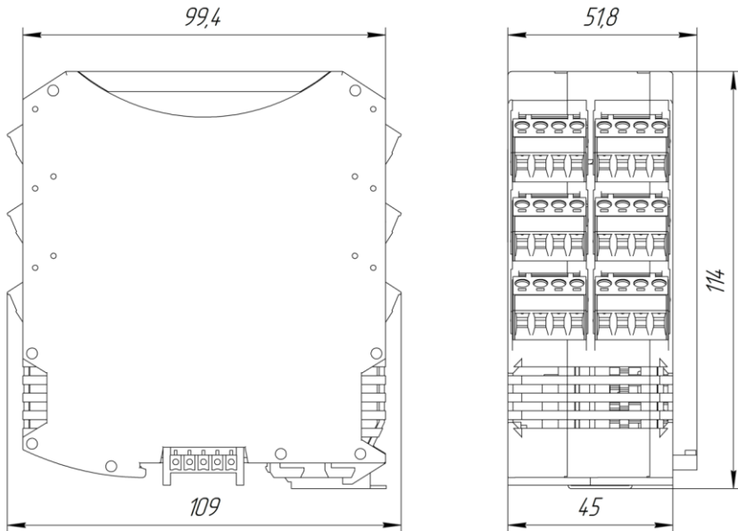
Рис. 1.15. Габаритный чертеж модуля
