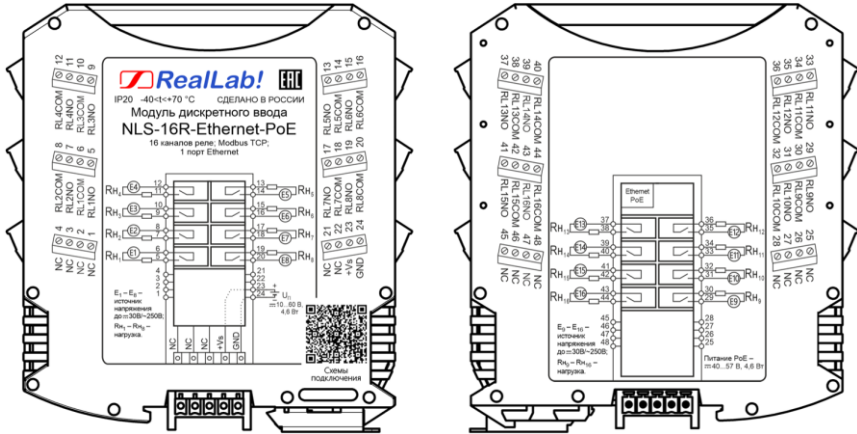
Рис. 1.12. Вид со стороны маркировки на модуль NLS-16R-Ethernet-PoE
