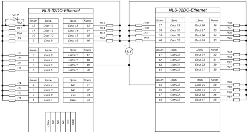
Рис. 4.24. Применение модулей NLS-32DO-Ethernet(-PoE), NLS-32DO-Ethernet-2P(-PoE) для управления нагрузкой, с питанием от одного внешнего источника
