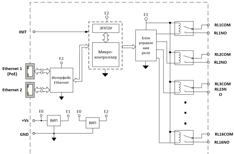
Рис. 3.8. Структурная схема модуля NLS-16R-Ethernet-2P(-PoE) Обозначения: COM - "Common" - "общий", "NO" - "Open" - нормально открытый
