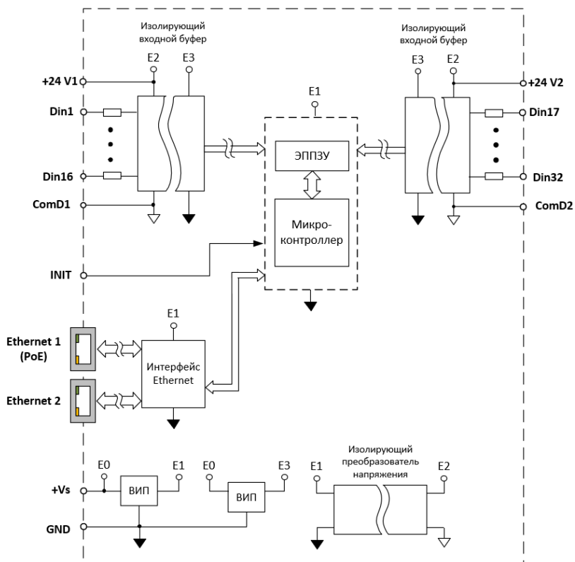
Рис. 3.2. Структурная схема модуля NLS-32DI-Ethernet-2P(-PoE)
