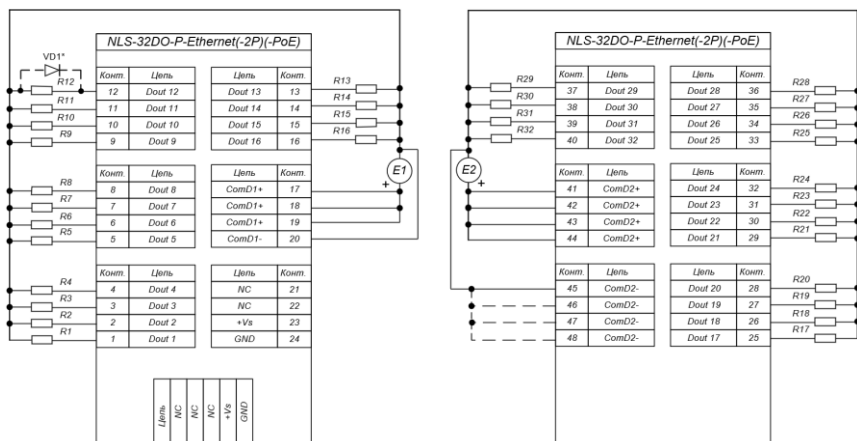
Рис. 4.25. Применение модулей NLS-32DO-P-Ethernet(-PoE), NLS-32DO-P-Ethernet-2P(-PoE) для управления нагрузкой, где:
