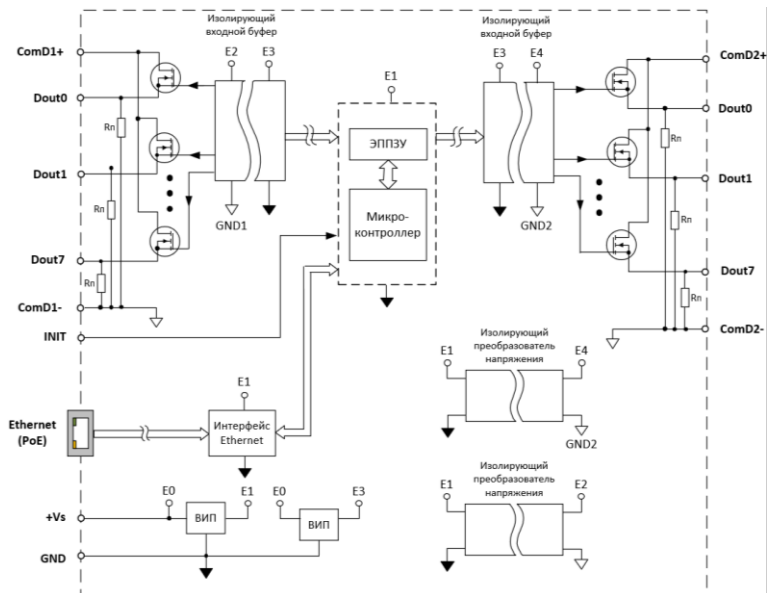
Рис. 3.5. Структурная схема модуля NLS-32DO-P-Ethernet(-PoE)
