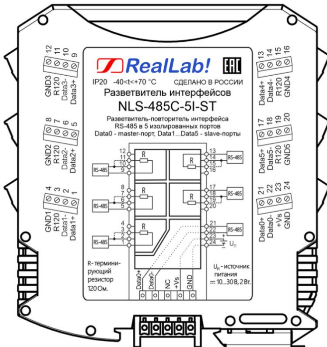
Рис. 1.2 Вид со стороны маркировки на модуль NLS-485C-5I-ST
