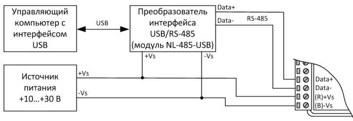
Рис. 4.4. Подключение модуля к порту RS-485 компьютера
