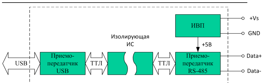
Рис. 3.2. Структурная схема модуля NL-485-USB-I-P
