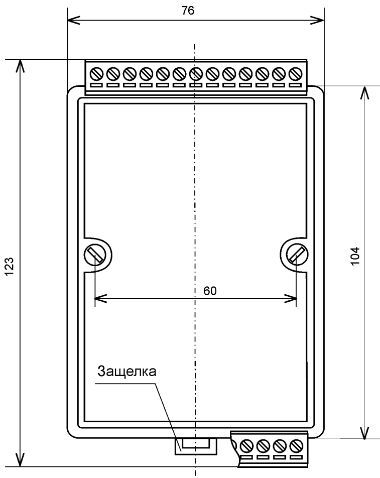
Рис. 1.3. Габаритный чертеж модуля.
