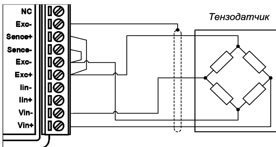
Рис. 6.1. Схема подключения тензодатчика к модулю по 4-х проводной схеме, без использования заземления
