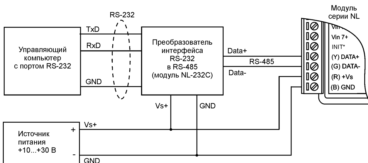
Рис. 6.7. Подключение модуля к порту RS-232 компьютера
