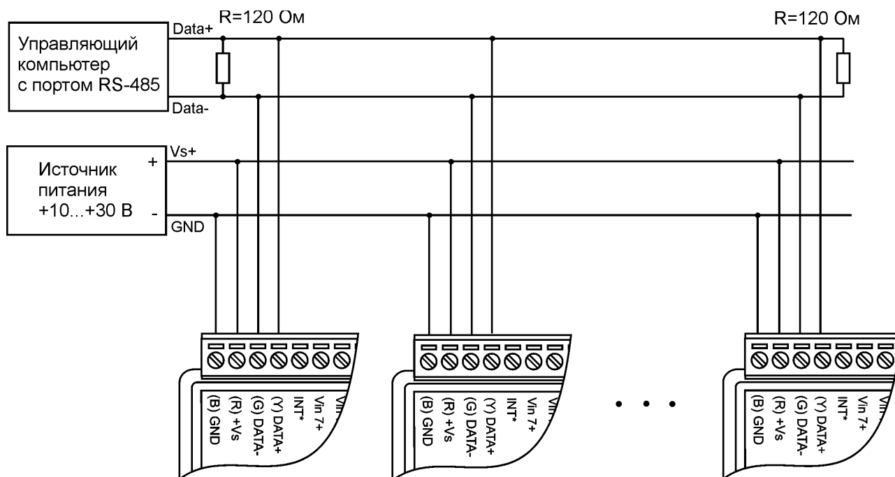
Рис. 6.9. Соединение нескольких модулей в сеть на основе интерфейса RS-485
