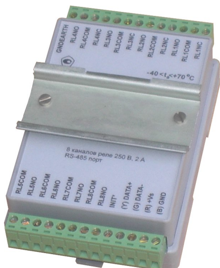
Рис. 6.4. Чтобы закрепить один модуль сверху другого, сначала закрепите ДИН-рейку сверху модуля.
