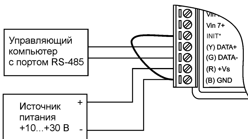
Рис. 6.8. Соединение вывода INIT* с "GND" для изменения скорости обмена и контрольной суммы
