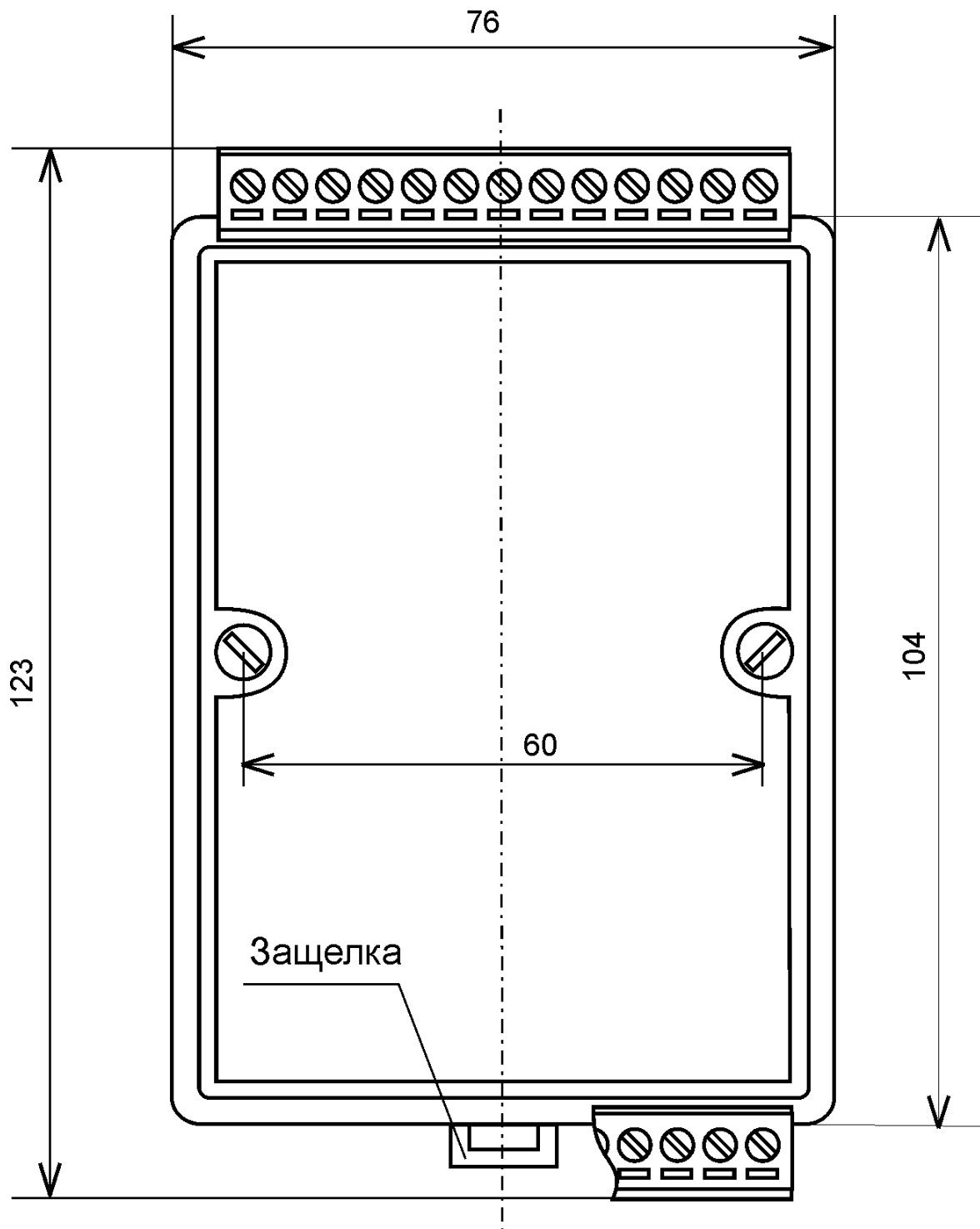
Рис. 2.2. Габаритный чертеж модуля.
