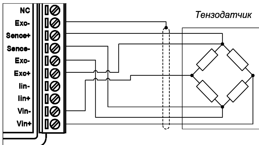
Рис. 6.3. Схема подключения нескольких тензодатчиков к модулю по 4-х проводной схеме, с использованием заземления
