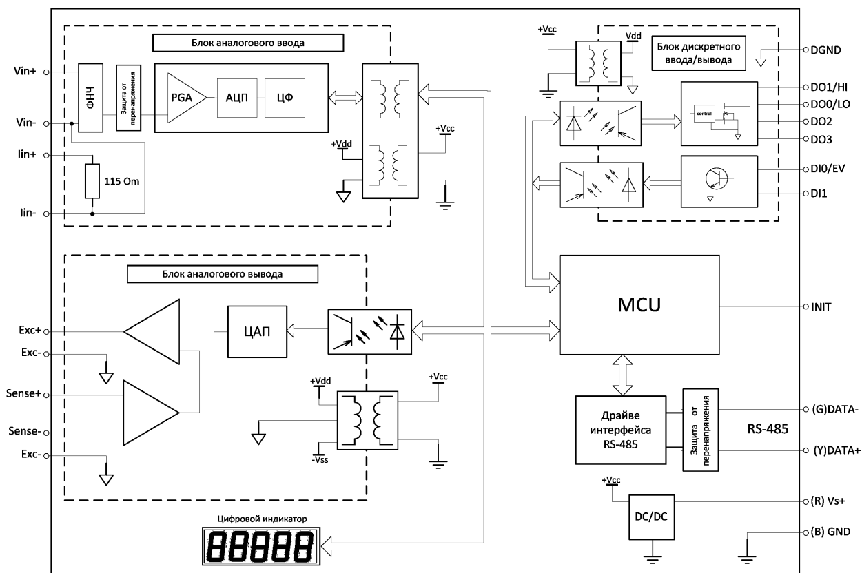
Рис. 4.1. Структурная схема модуля
