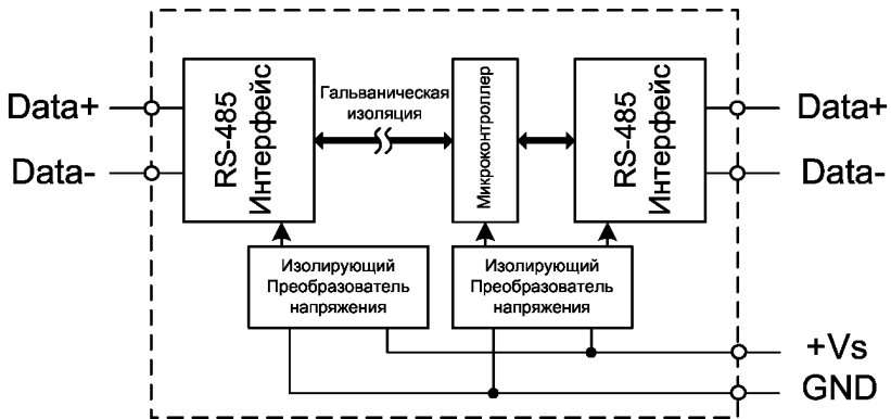
Рис. 3.1. Структурная схема модуля NL-485C-Ex
