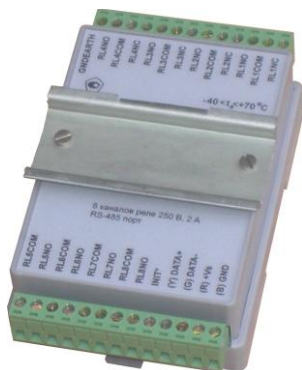
Рис. 4.3. Чтобы закрепить один модуль сверху другого, сначала закрепите ДИН-рейку сверху модуля.
