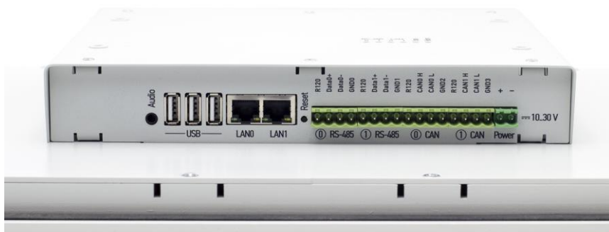
Рис. 1.4 Панельный ПЛК NLcon-LXD18, вид снизу
