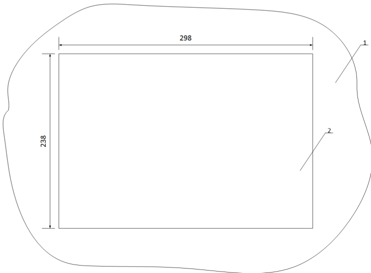
1 – Монтажная панель 2 – Отверстие для монтажа NLcon-CED12
