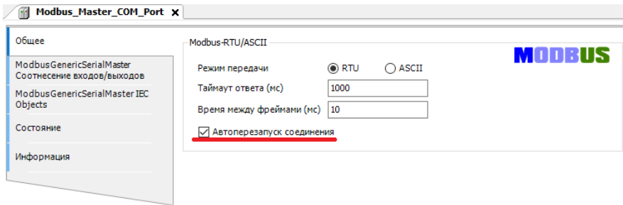
Рис. 4.14. Настройки Modbus Master COM Port
