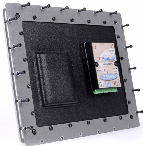
Рис. 1.2. Панельный ПЛК NLCon-CED12, вид сзади
