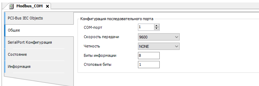
Рис. 4.22. Настройки Modbus COM
