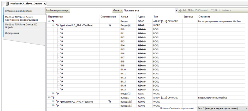
Рис. 4.42. Соотнесения каналов и переменных Slave-устройства
