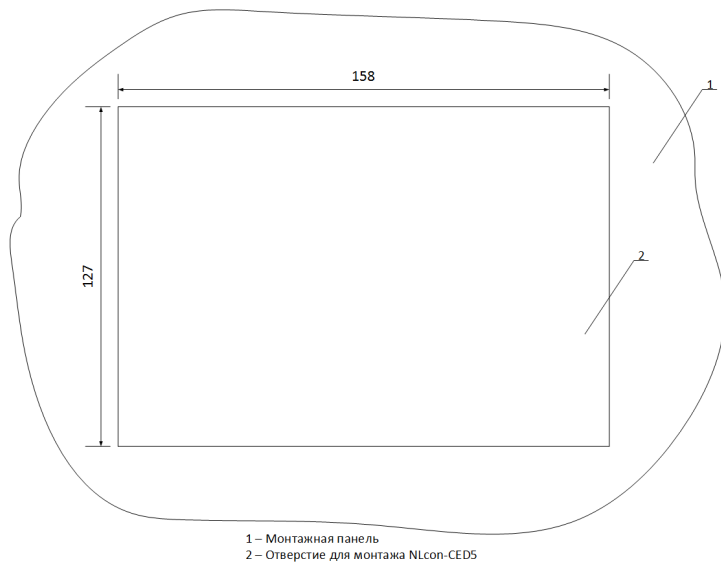
Рис. 4.1. Монтажное отверстие для NLCon-CED5
