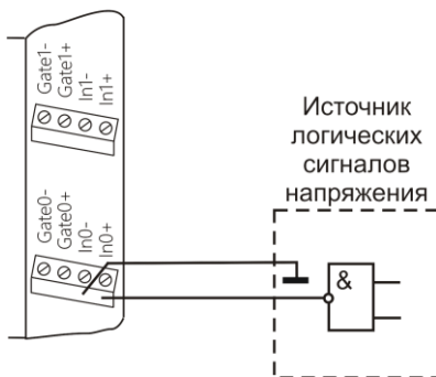
Рис. 6.5. Подключение источников логических сигналов к модулю. Входы разрешения счета не используются
