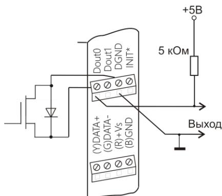
Рис. 6.8. Получения логических уровней напряжения на выходах модуля
