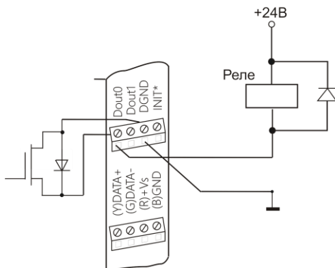
Рис. 6.7. Применение модуля для управления электромагнитным реле
