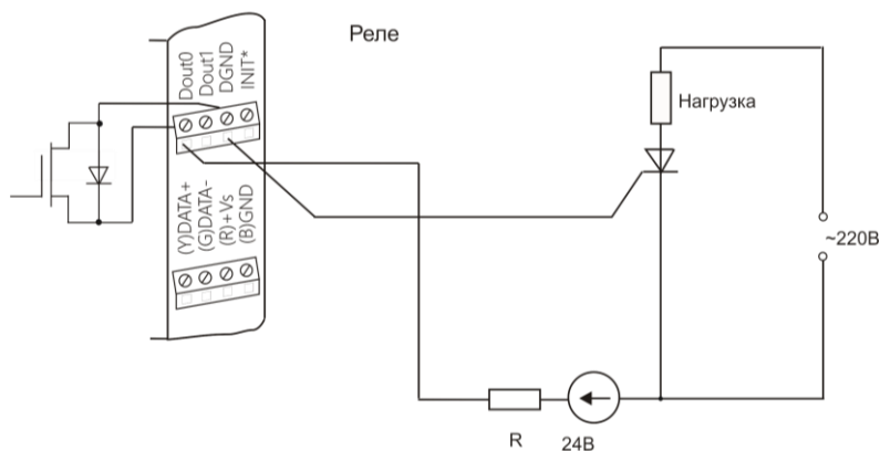
Рис. 6.6. Применение модуля для управления мощным тиристором
