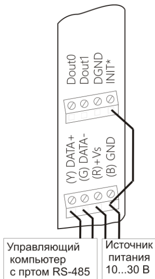
Рис. 6.4. Соединение вывода “INIT” с "землей"
