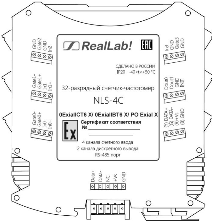
Рис. 2.1 Вид со стороны маркировки на модуль NLS-4C взрывозащищенного исполнения
