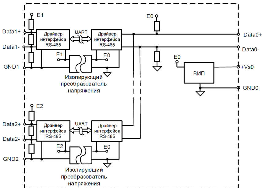
Рис. 3.1 Структурная схема модуля NLS-485C-Ex взрывобезопасного исполнения
