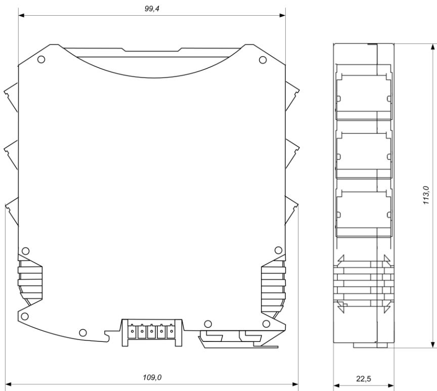
Рис. 1.3. Габаритный чертеж модуля.
