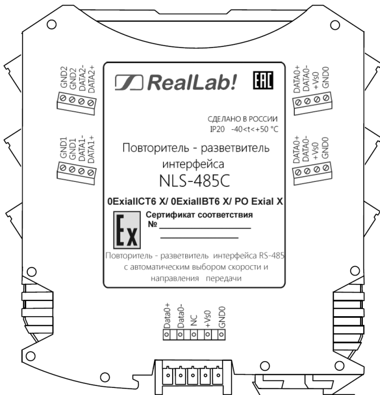
Рис. 1.1 Вид со стороны маркировки на модуль NLS-485C-Ex взрывозащищенного исполнения
