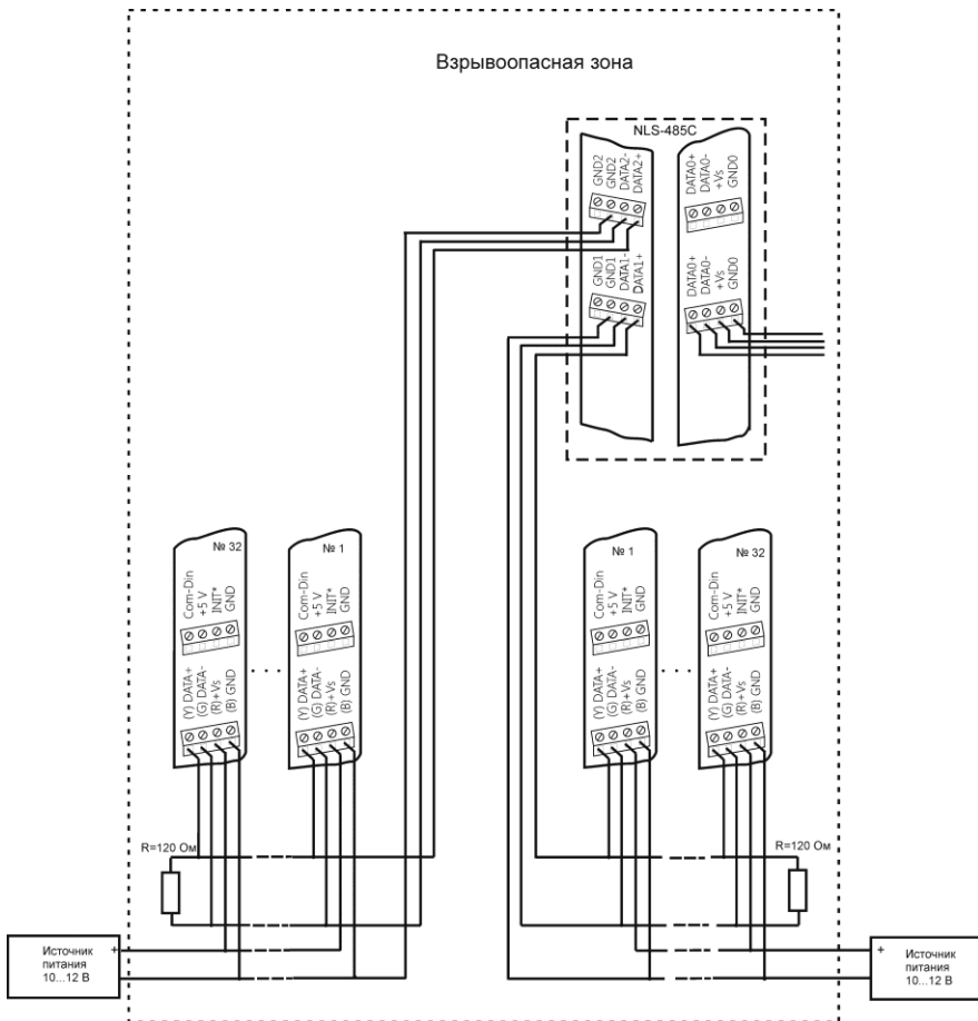
Рис. 4.4. Подключение модулей серии NLS в секционированную сеть на основе интерфейса RS-485
