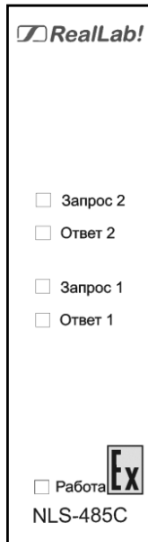
Рис. 4.1. Расположение органов индикации на лицевой панели модуля NLS-485C-Ex взрывобезопасного исполнения
