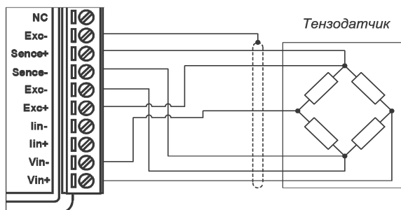
Рис. 6.3. Схема подключения нескольких тензодатчиков к модулю по 4 х проводной схеме, с использованием заземления
