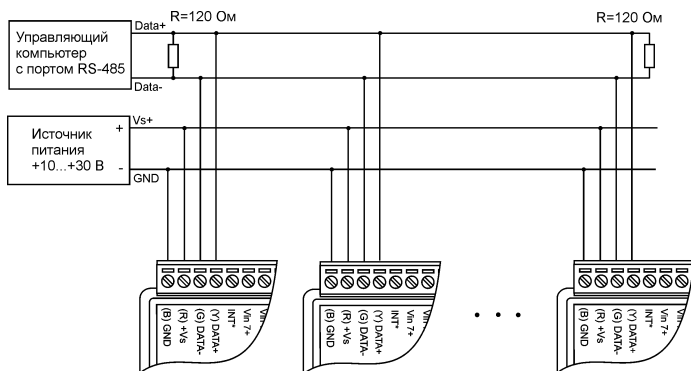
Рис. 6.9. Соединение нескольких модулей в сеть на основе интерфейса RS-485
