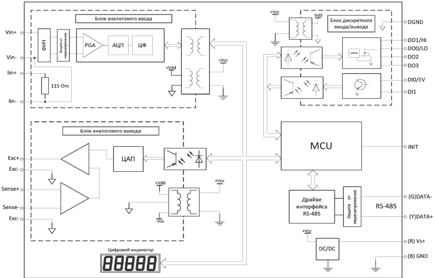
Рис. 4.1. Структурная схема модуля NLS-4AO
