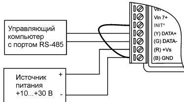
Рис. 6.8. Соединение вывода INIT* с "GND" для изменения скорости обмена и контрольной суммы
