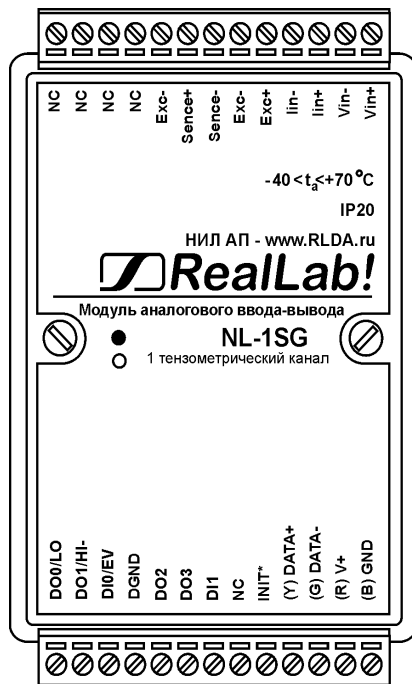
Рис. 2.1. Внешний вид на модуль NL-1SG. Вид сверху
