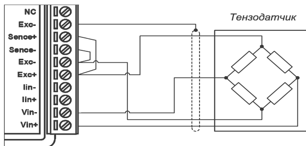
Рис. 6.1. Схема подключения тензодатчика к модулю по 4-х проводной схеме, без использования заземления
