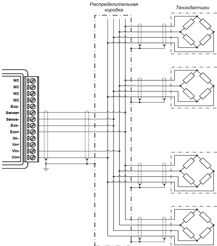
Рис. 6.2. Схема подключения тензодатчика к модулю по 6-ти проводной схеме, без использования заземления
