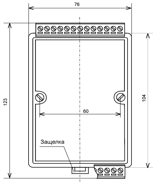
Рис. 2.2. Габаритный чертеж модуля
