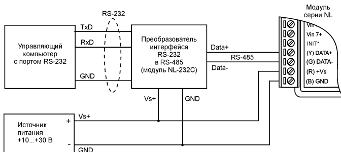
Рис. 6.7. Подключение модуля к порту RS-232 компьютера
