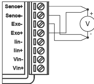
Рис. 5.1. Соединение приборов для юстировки источника напряжения возбуждения
