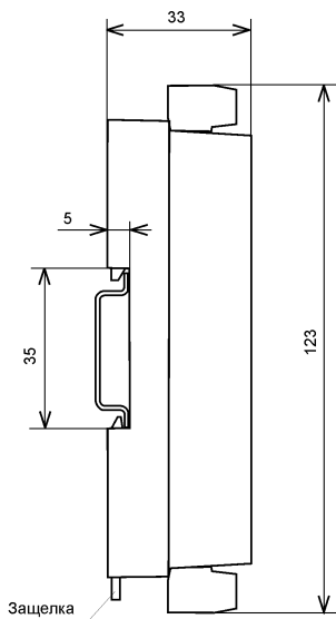
Рис. 2.3. Габаритный чертеж модуля
