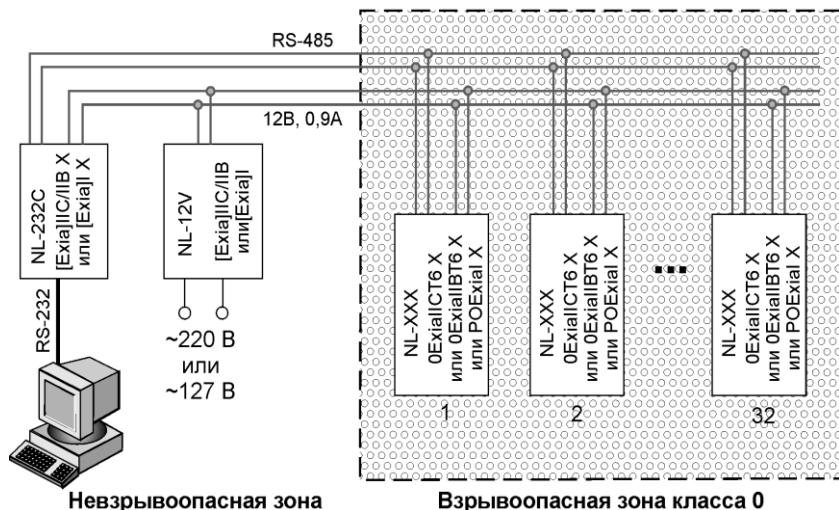
Рис. 6.1. Блок-схема искробезопасной системы на плане взрывоопасных зон
