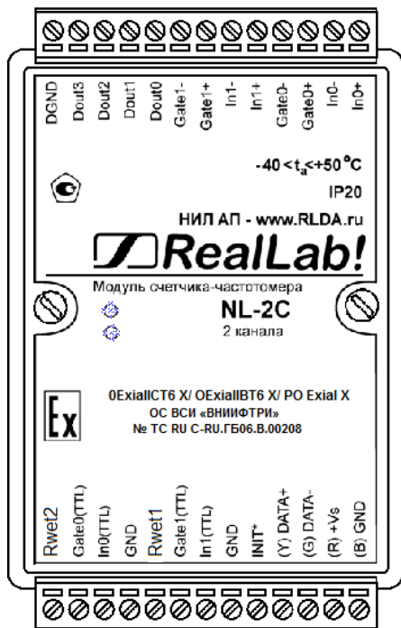
Рис. 2.1. Вид сверху на модуль NL-2C, взрывозащищённого исполнения
