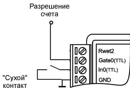
Рис. 6.5 . Подключение источника дискретных сигналов типа "сухой контакт" к модулю NL-2С, взрывозащищённого исполнения
