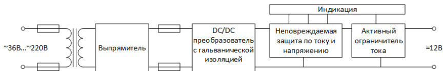
Рис. 3.1. Структурная схема источника питания
