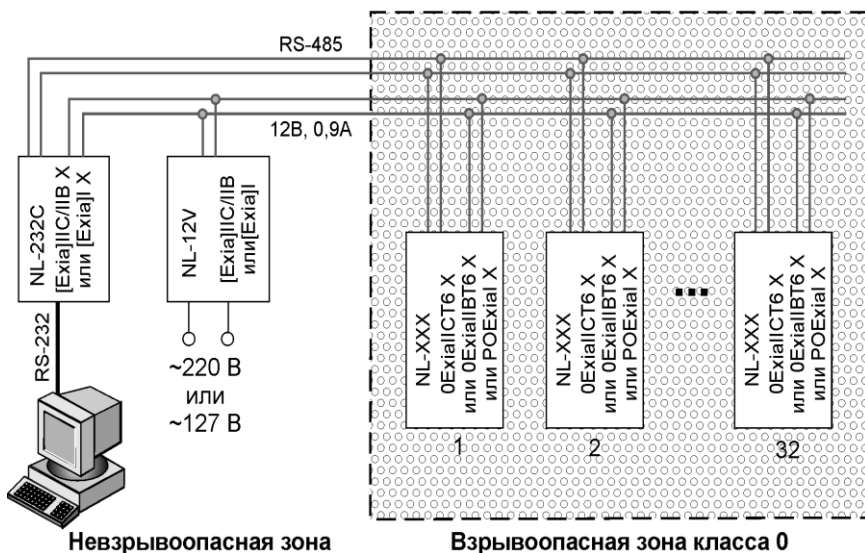
Рис. 4.1. Блок-схема искробезопасной системы на плане взрывоопасных зон
