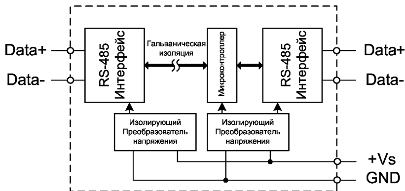
Рис. 3.1. Структурная схема модуля NL-485C
