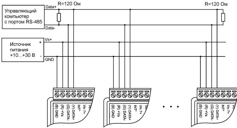
Рис. 4.5. Соединение нескольких модулей в сеть на основе интерфейса RS-485
