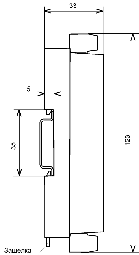
Рис. 1.4. Габаритный чертеж модуля с креплением к DIN-рейке. Вид сбоку
