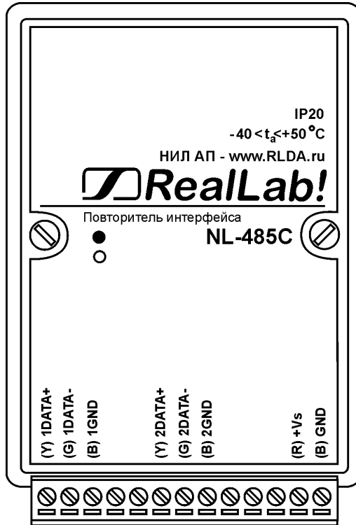
Рис. 1.2. Вид сверху на модуль NL-485C
