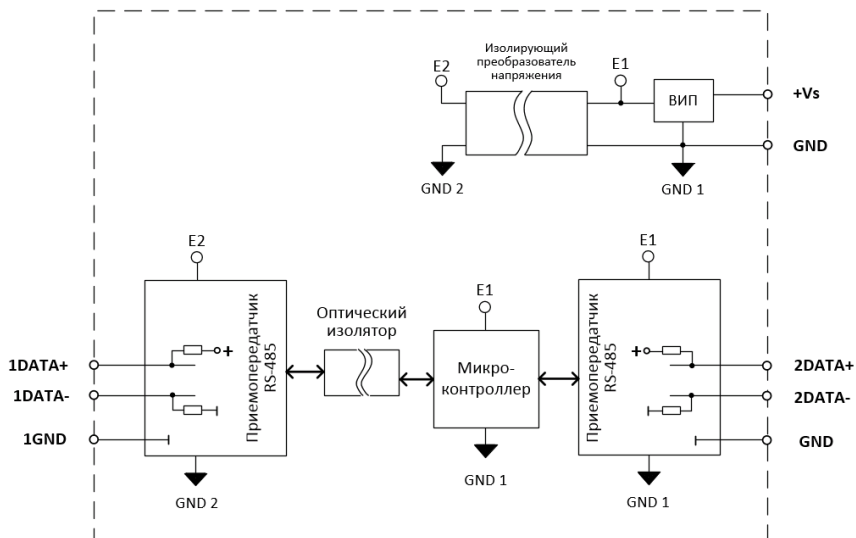
Рис. 3.3. Структурная схема модуля NL-485C-2
