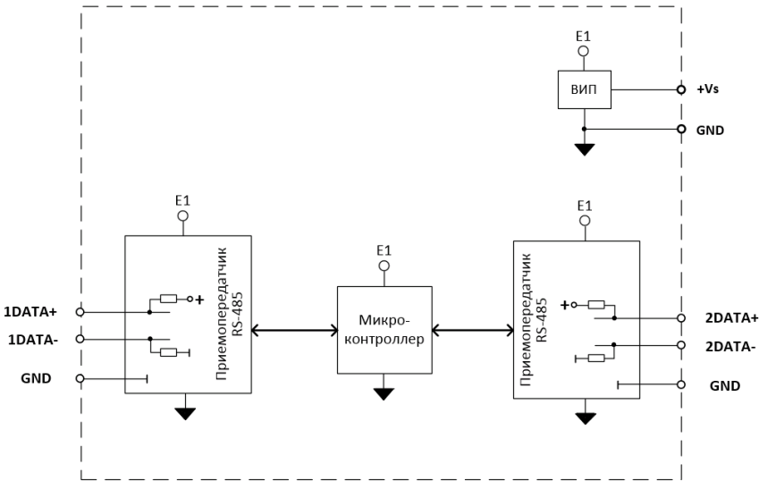
Рис. 3.2. Структурная схема модуля NL-485C-1
