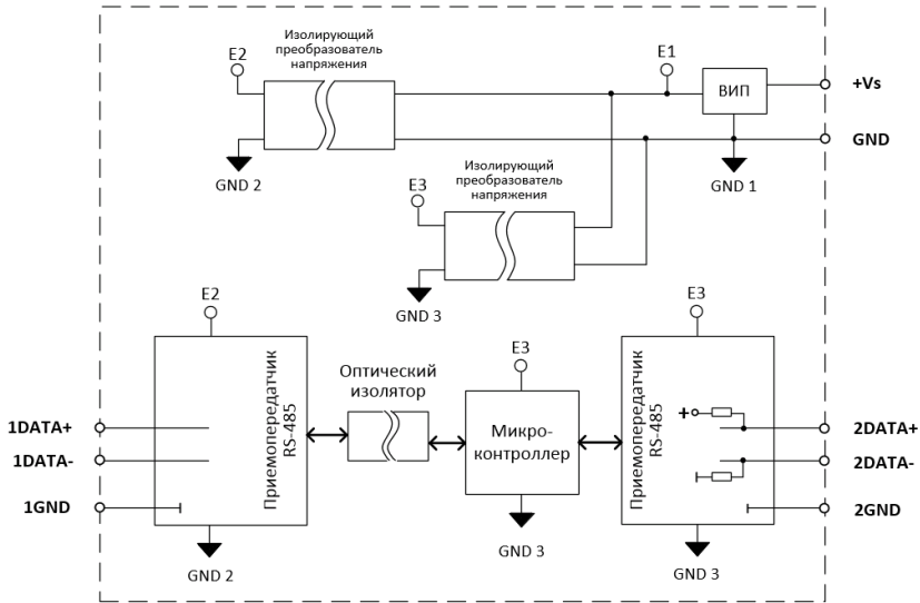
Рис. 3.5. Структурная схема модуля NL-485C-4
