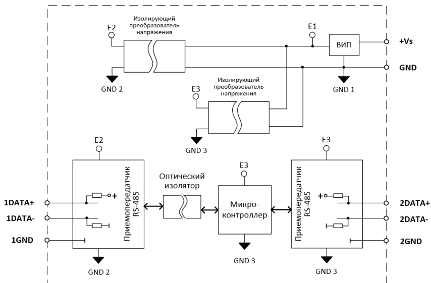
Рис. 3.4. Структурная схема модуля NL-485C-3
